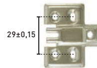
Calço SPM 175°
