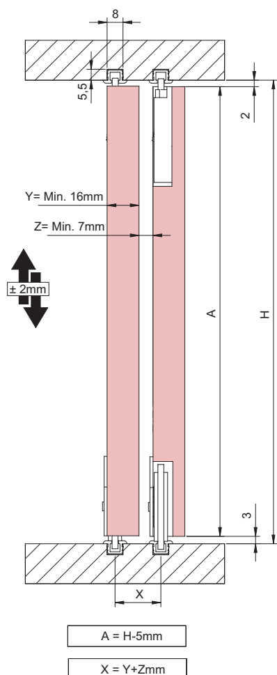
Instalação com roldanas / acessórios encastrados
