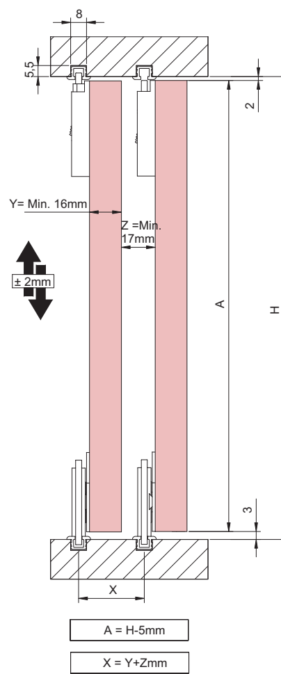
Instalação com roldanas / acessórios sobrepostos
