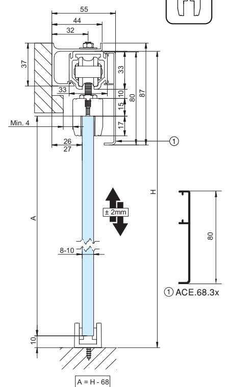
Instalação na parede com perfil separador
