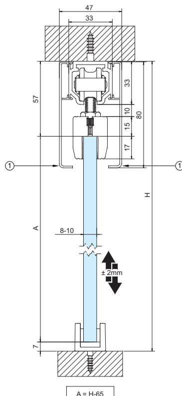
Instalação no tecto
